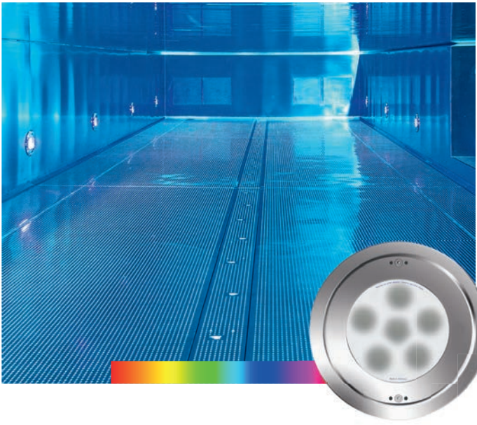
Projecteurs immergés à LED
